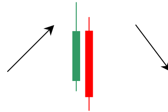
Tweezer Top
