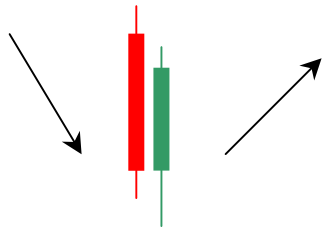
Tweezer Bottom
